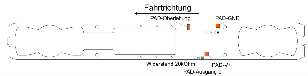
Abbildung 2: Rahmenplatte Ansicht von oben
