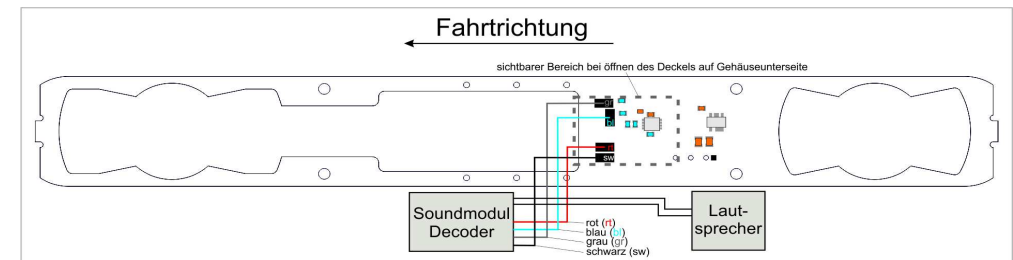
Abbildung 1: Rahmenplatte Ansicht von unten (Montage SUSI-Soundmodul)
